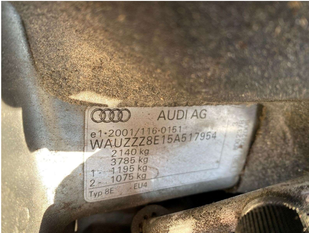
Bild: 29 Typenschild mit Fahrzeugidentnummer
