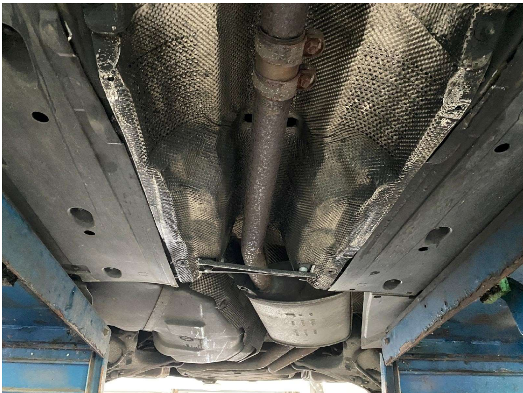
16 diverse Streifbeschädigungen am Unterboden hinten
