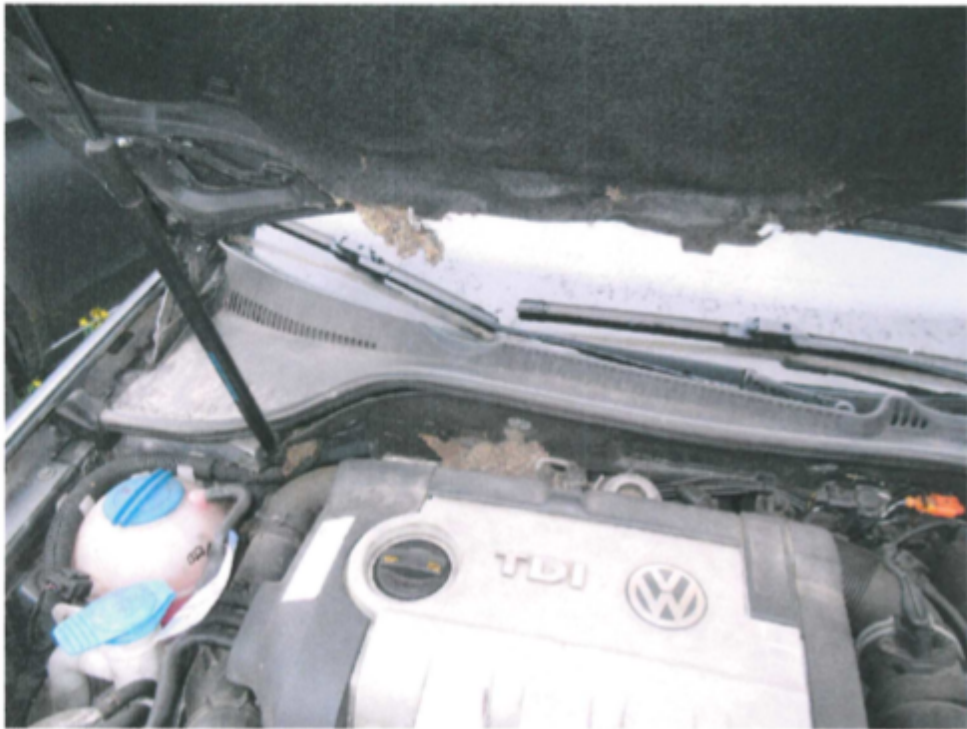
Bild 9 : Motorhaubendämmmatte zerfressen
