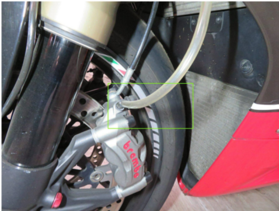
Bild 11 : Bremsanlage vorn nicht ordnungsgemäßer Zustand
