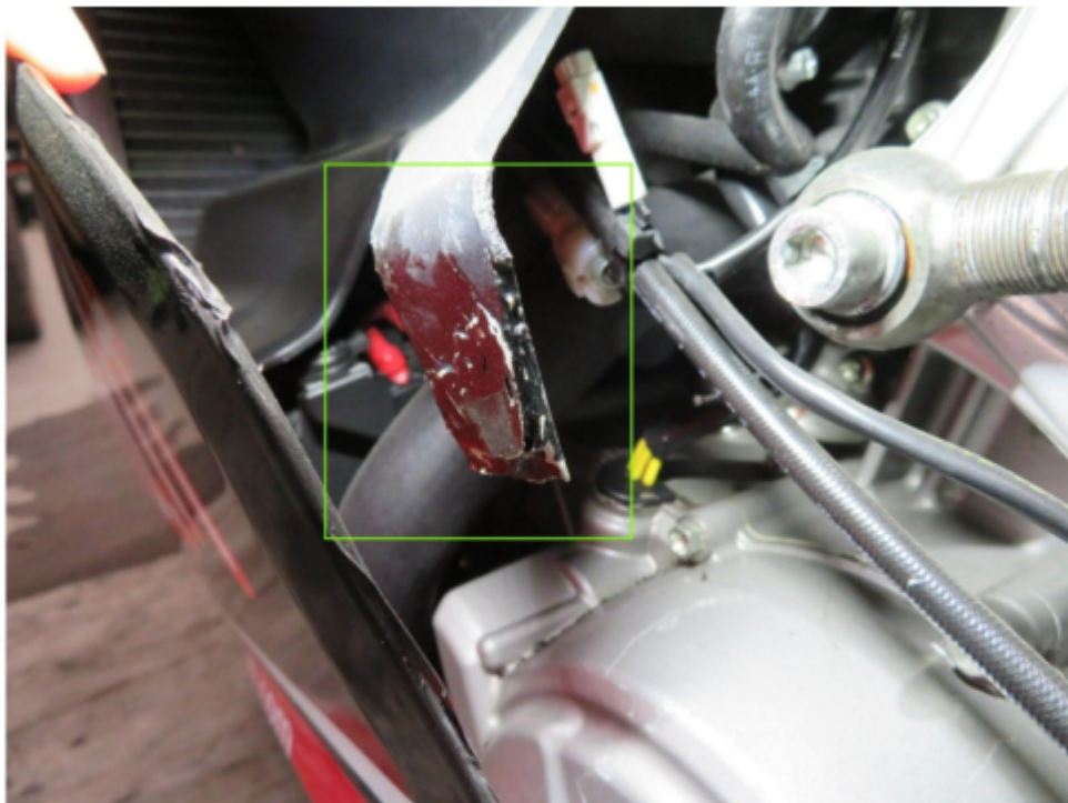
Bild 16 : Halterung Seitenverkleidung gebrochen
