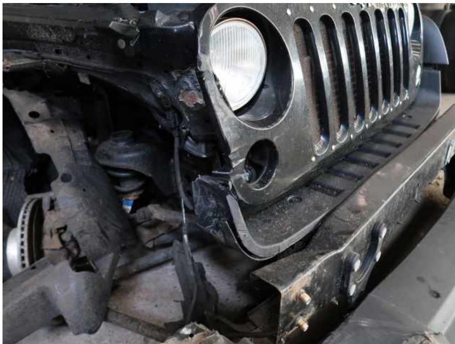
Verformter Kühlergrill und Querträger
