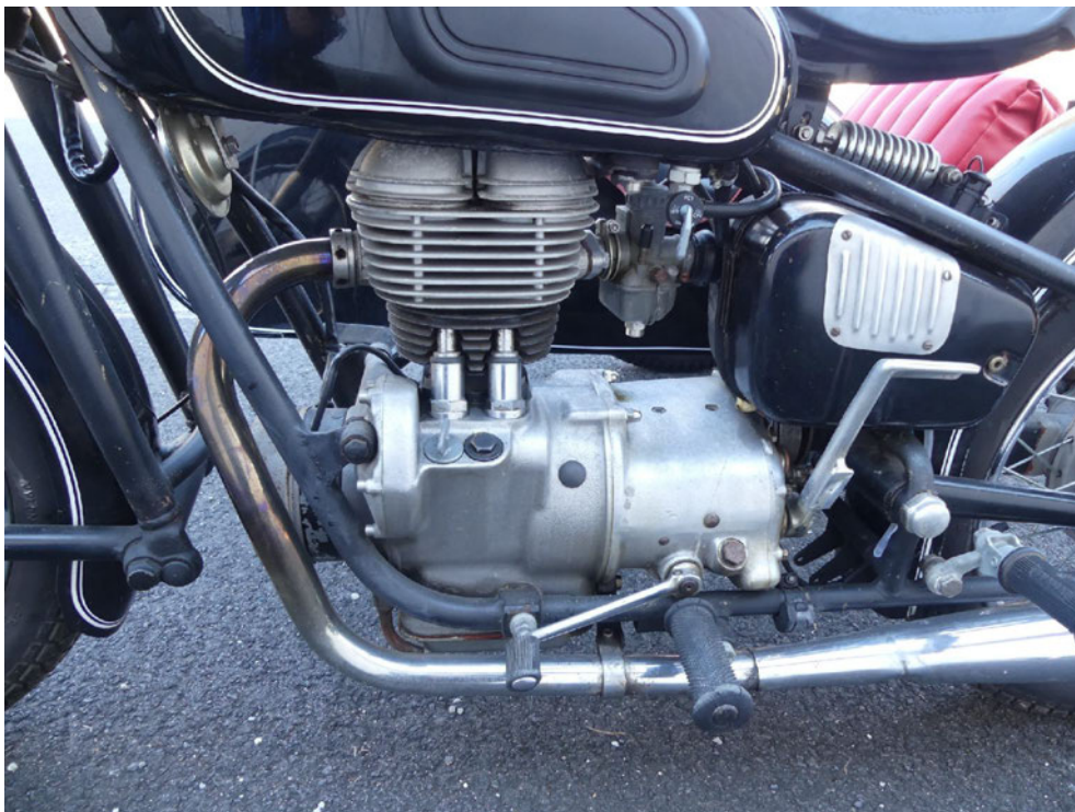
Bild: 12 Detailansicht Motor
