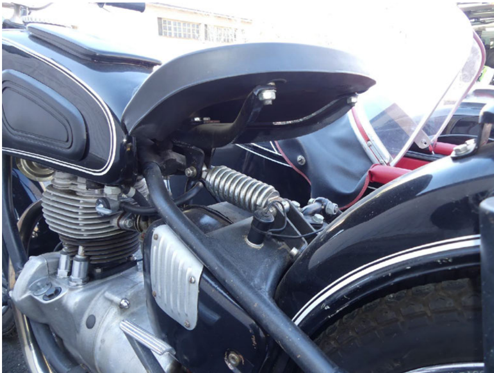
Bild: 15 Weitere Detailansicht Fahrersitz.
