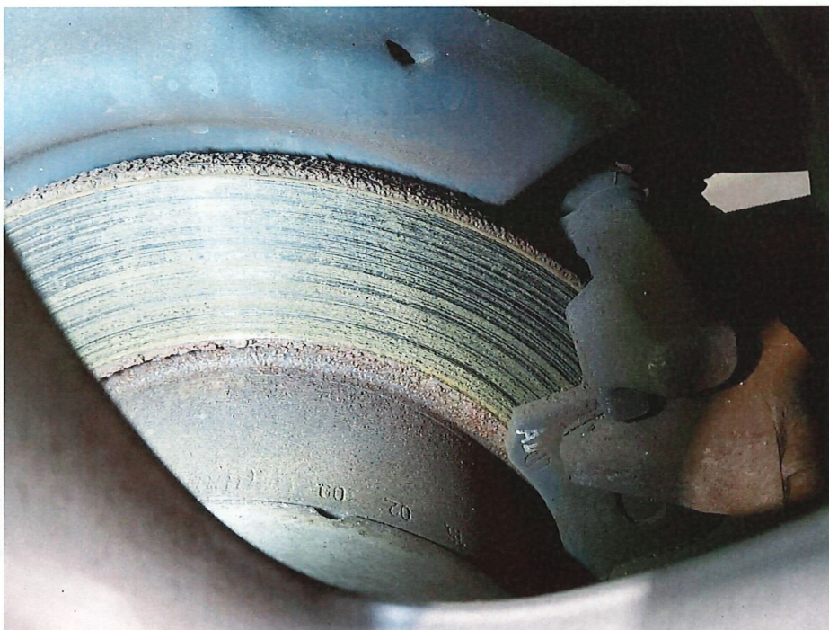
Bild 10 : Bremsscheiben angerostet
