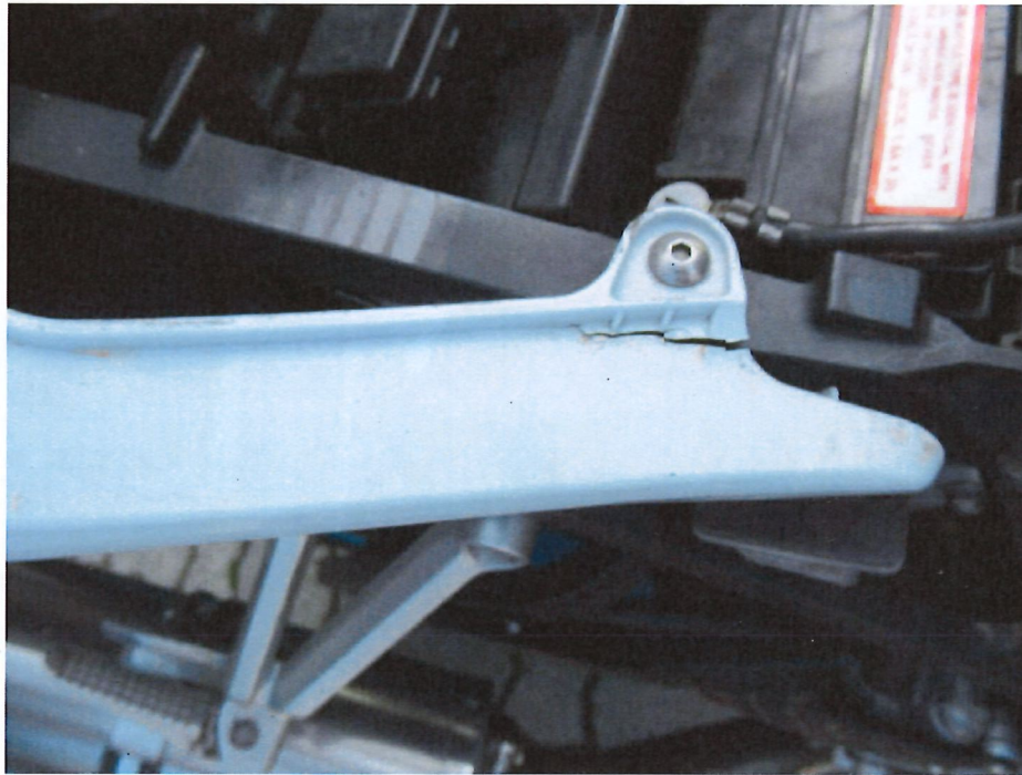
Bild 17 : Heckverkleidung gebrochen
